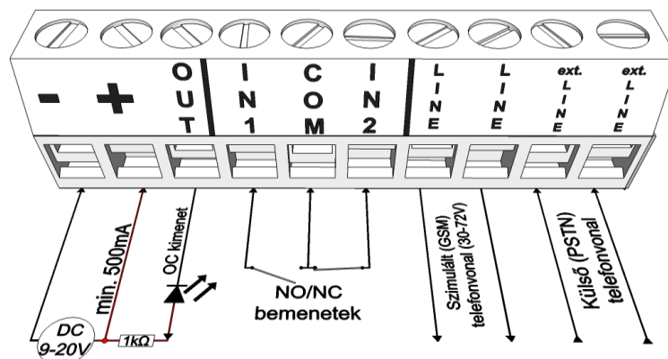
3. ábra: A sorkapocs bekötési sorrendje
