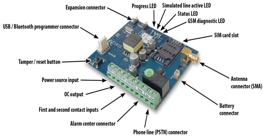
2. ábra: a modul felépítése
