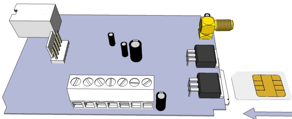
3. ábra SIM kártya behelyezése
